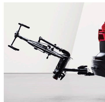
FOLDING BICYCLE HOLDER FOR TOWBAR, 2 BICYCLES - FIX4BIKE น้ำหนักเบา และติดตั้งง่าย ยึดกับตะขอลากจูง สำหรับจักรยาน 2 คัน *48,500 บาท* (P/N: 32296829)
